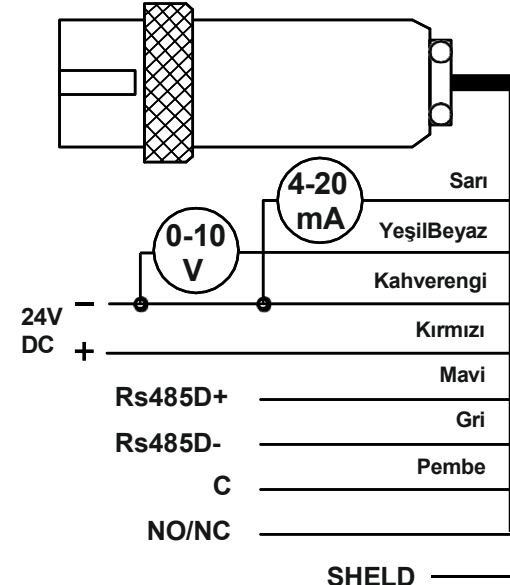
ENCO-101 MIKE KONNEKTÖR
