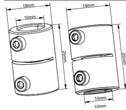
10x10mm Esnek kaplin
