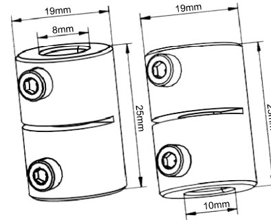
10x8mm Esnek kaplin
