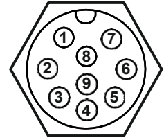
ENCO-102 MIKE KONNEKTÖR
